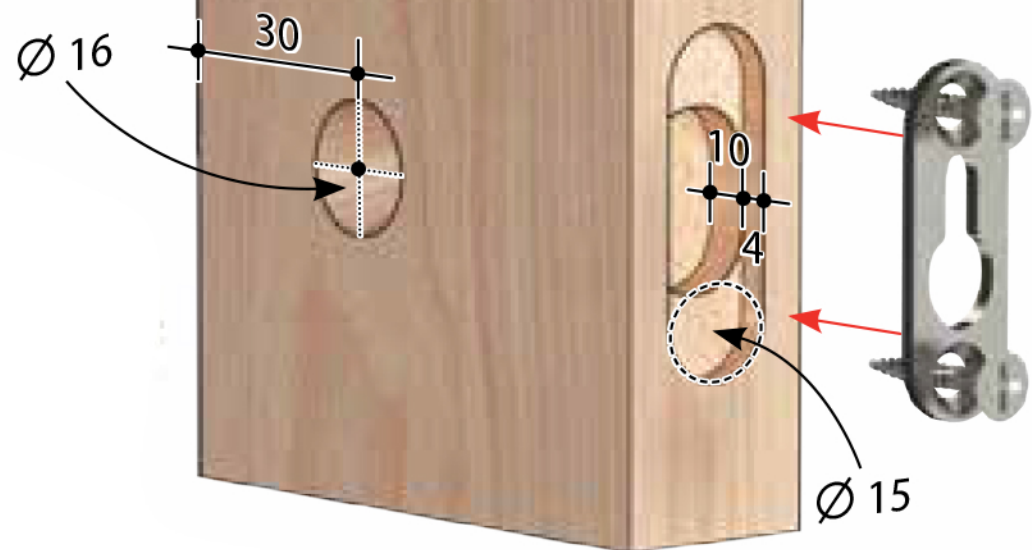
Wandbefestigung
